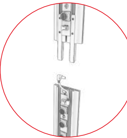
Led Bağlantı | Led Connection
