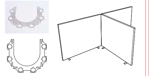
T Bağlantı Aparatı / T Shape Connector
