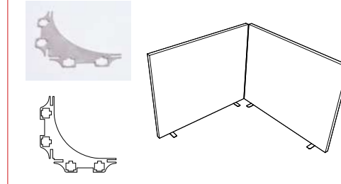
L Bağlantı Aparatı / L Shape Connector
